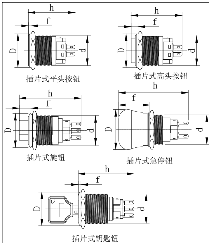
图二:产品外形尺寸图
