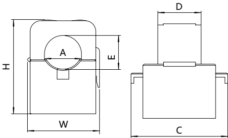
ALH-0.66SK*L 型
