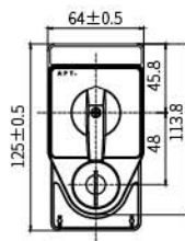
标牌框带钥匙型 LW39-25 PYM-□-□/□□□□
