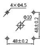
客户安装开孔尺寸
