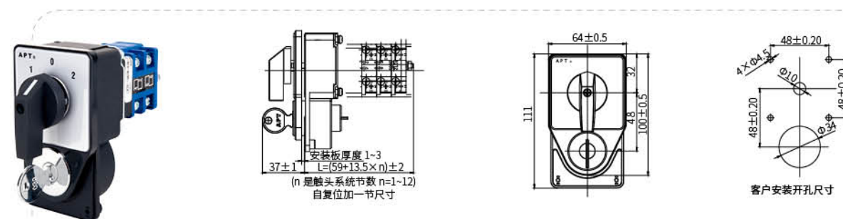
面板钥匙型 LW39-16NYM-□-□...□/□-□-□-□...□-□
