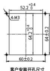
客户安装开孔尺寸
