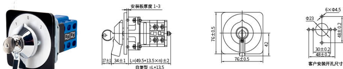
手柄带钥匙型 LW39-25 YS-□-□/□□□
