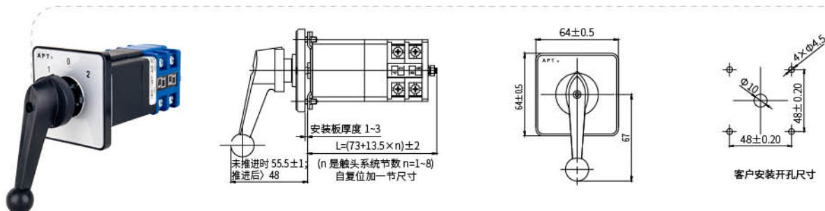
一般推进（拉出）型 LW39-16NTF(LF)/TC(LC) -□-□...□/□-□-□-□...□-□
