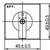
三孔安装型LW39-16B S-□-□/□□□
