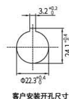
客户安装开孔尺寸
