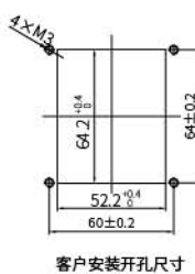
客户安装开孔尺寸
