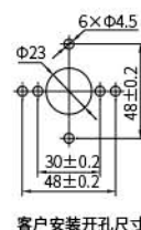
手柄带钥匙型 LW39-63 YS-□-□/□□□
