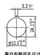
一般型LW39-16C-□-□/□□
