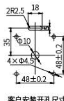
客户安装开孔尺寸
