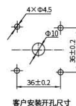
一般型 LW39-16B-□-□/□□□
