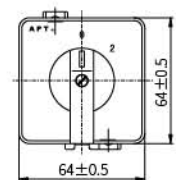
底座安装型 LW39-25 M-□-□/□□□
