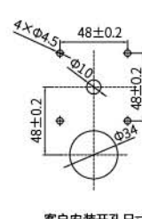
客户安装开孔尺寸
