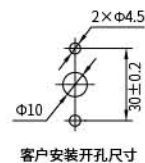
三孔安装型LW39-16B S-□-□/□□□
