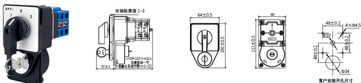
面板带钥匙型 LW39-25 YM-□-□/□□□
