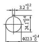
客户安装开孔尺寸
