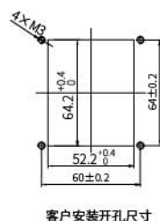
客户安装开孔尺寸
