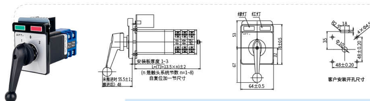
带灯推进（拉出）型 LW39-16NTFD(LFD) -□-□...□/□-□-□-□...□-□
