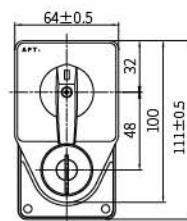
面板带钥匙型LW39-16B YM-□-□/□□□
