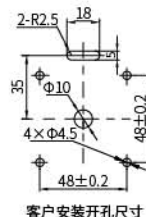
面板带灯型 LW39-63 DM-□-□/□□□□
