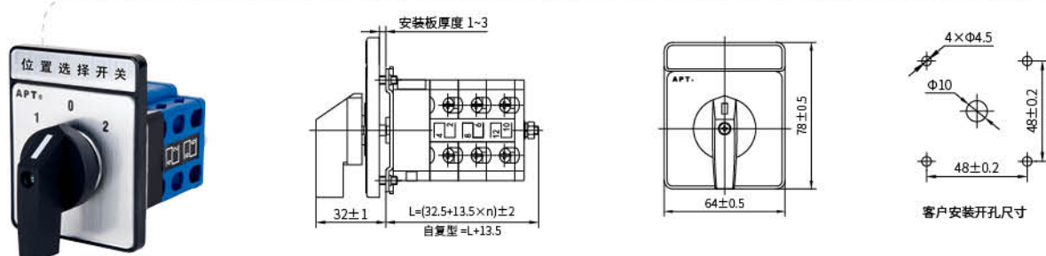
带标牌型 LW39-25 P2-□-□/□□□
