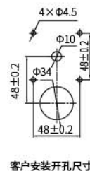
面板带钥匙型LW39-16B YM-□-□/□□□
