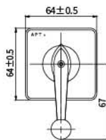
拉出（推进）操作型 LW39-25 LC (TC) -□-□/□□□□
