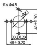
客户安装开孔尺寸
