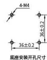
底座安装型 LW39-16B M-□-□/□□□
