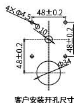
客户安装开孔尺寸
