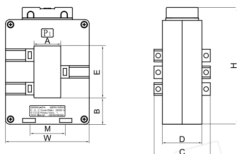
ALH-0.66 III型
