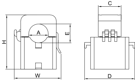
ALH-0.66 SK10/16/24/36L 型
