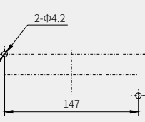
箱体安装开孔尺寸图
