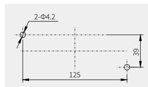
箱体安装开孔尺寸图
