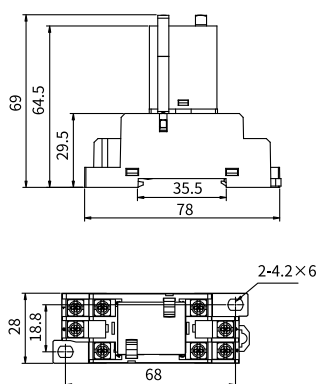
A3 型 (仅用于 STF11A 和 STF14A)
