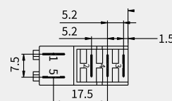
安装孔尺寸
