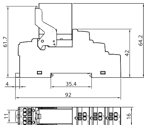
SR1ML 继电器 + SSP05F 插座
