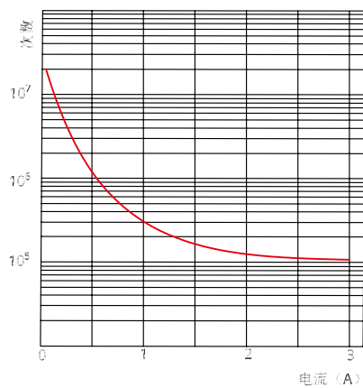
HR4C 阻性负载
