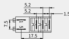
安装孔尺寸
