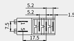
安装孔尺寸
