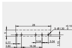
安装孔尺寸
