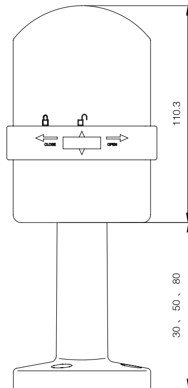
外型尺寸
