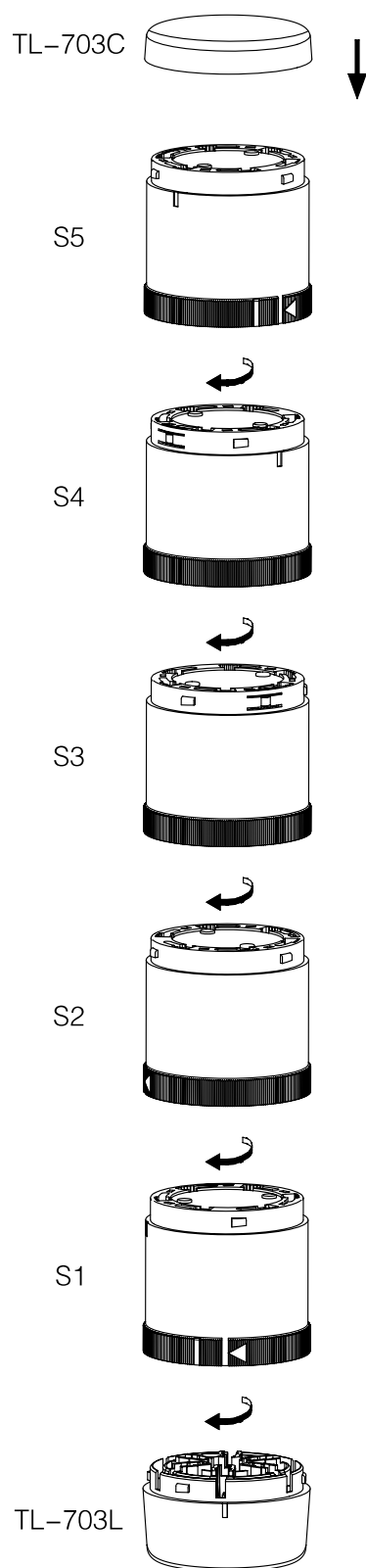
安装示意图
