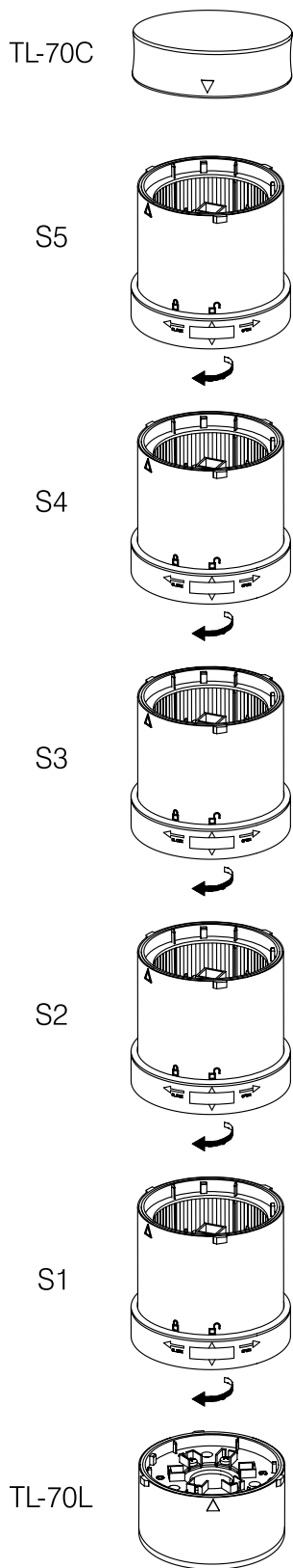
安装示意图
