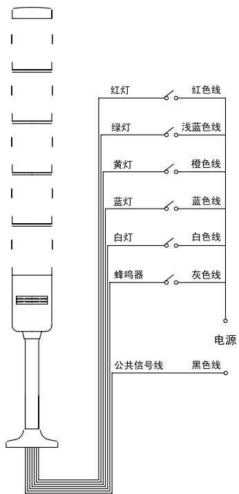
常亮型
