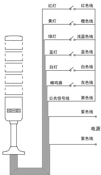
闪亮型
