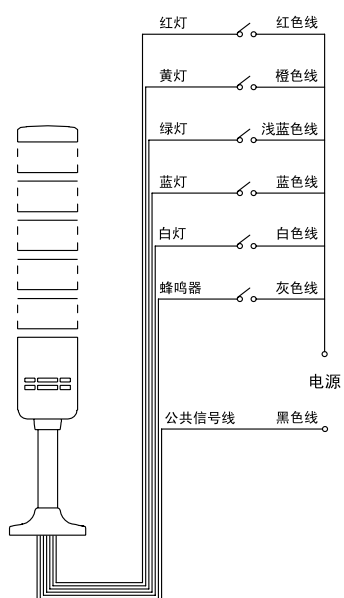
常亮型
