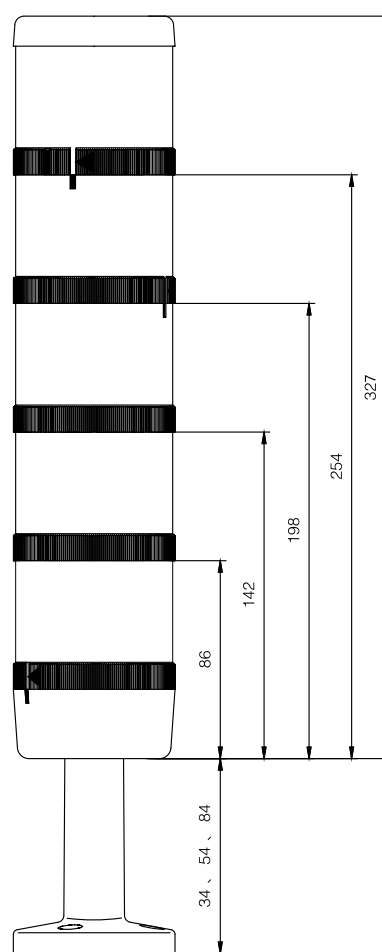
外型尺寸
