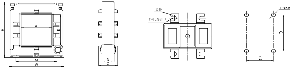
ALH-0.66 HK型
