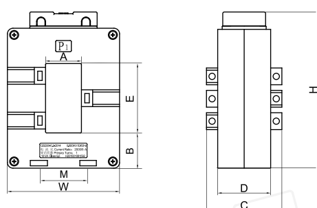
ALH-0.66 III型
